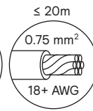
RS-485 DyNet SELV/Class 2 (UL)
